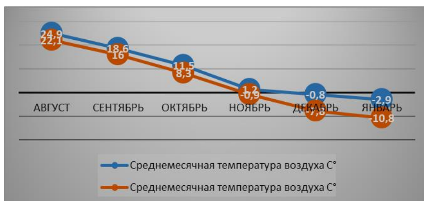
Рисунок 3 – Среднемесячная температура осенне-зимнего периода 2019-2020 гг. в Алматинской области
