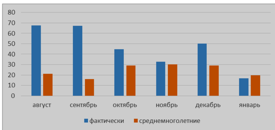
Рисунок 2 – Среднемесячное количество осадков осенне-зимнего периода 2019 г. в Алматинской области
